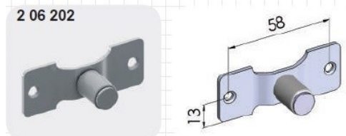
2 06 202 HMR AKS orta kapak destek elemanı HMR AKS Center platform support element Элемент для поддержки средней плиты
