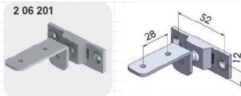
2 06 201 HMR AKS Orta kapak hareket kapalı mili ve plastiği HMR AKS Center platform moving pin-closed Подвижная Ось для Средней Плиты-закрытая
